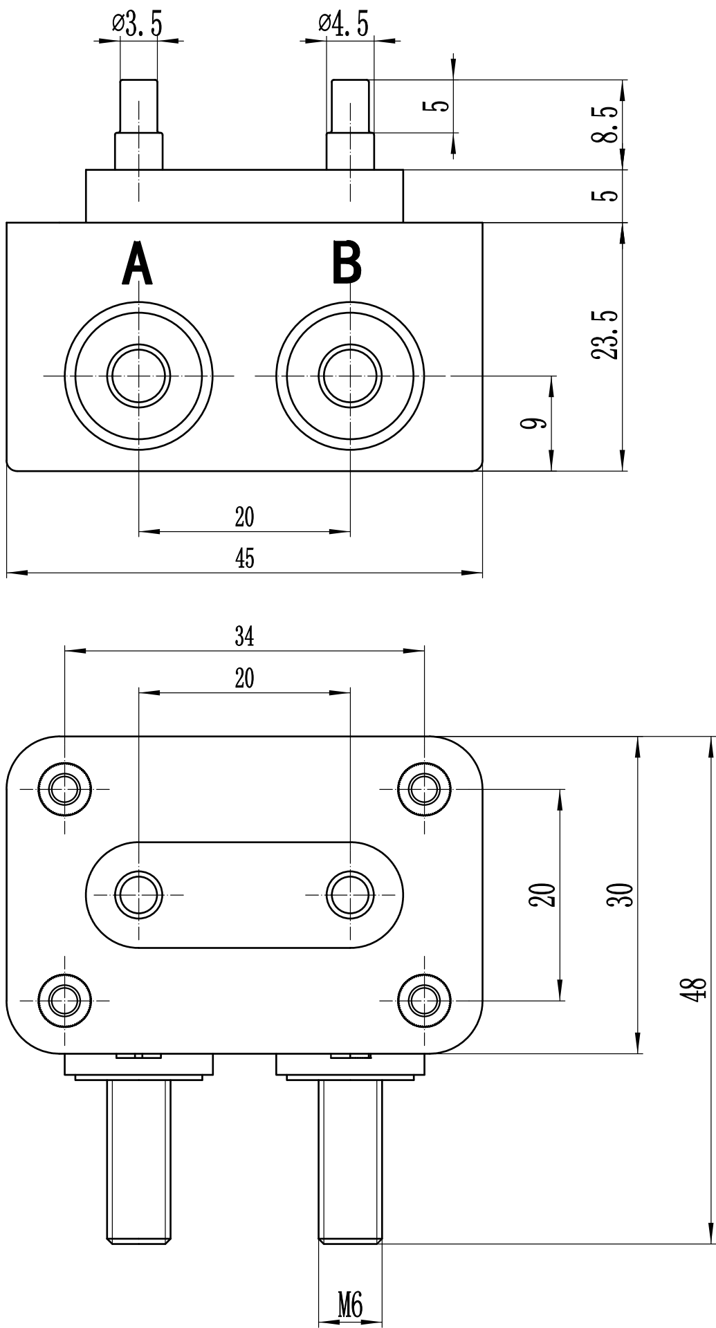
DZ-AB 二芯短路端子
